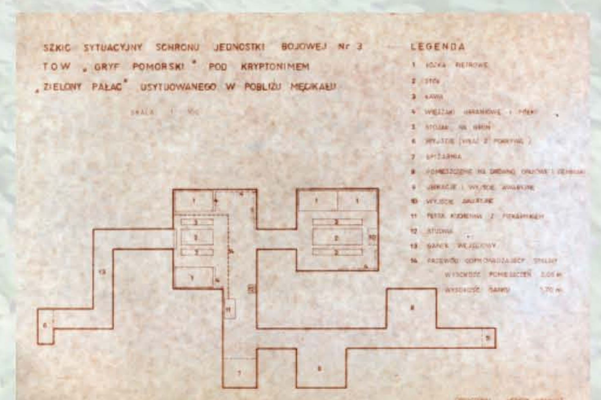
Plan inwentaryzacji bunkra TOW „Gryf Pomorski” kryptonim „Zielony Pałac” (AMS)
